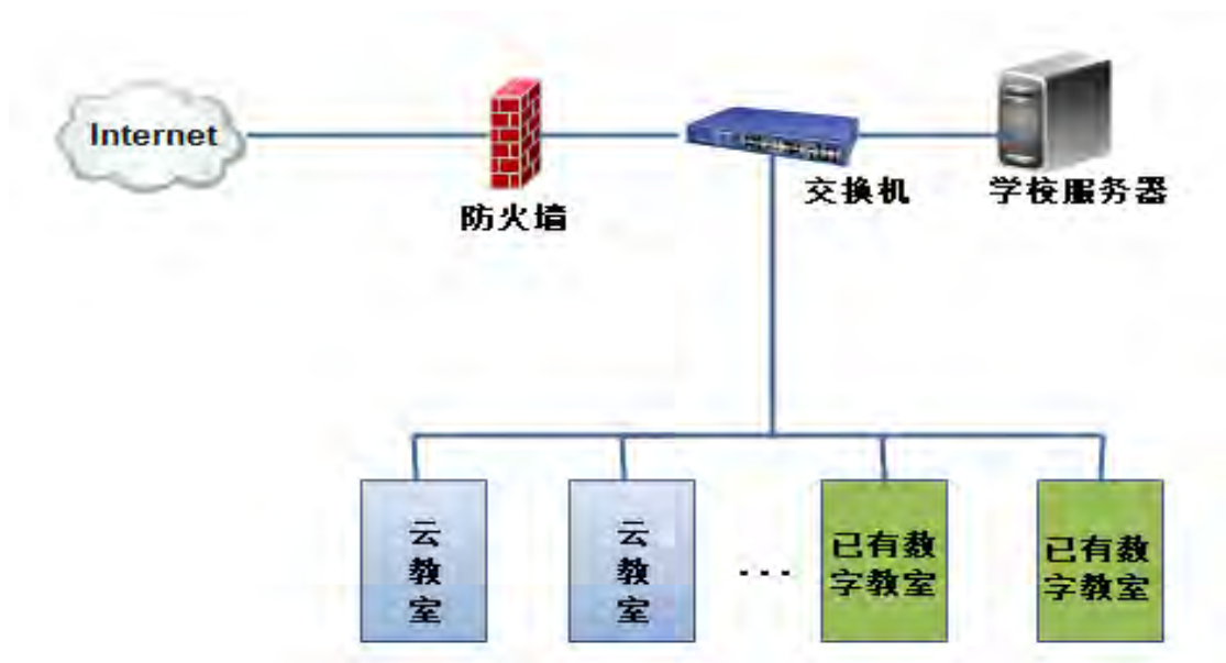
图13-7 云校园网络架构图
